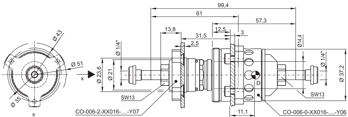
Einbaubeispiel / Installation example DN 6
