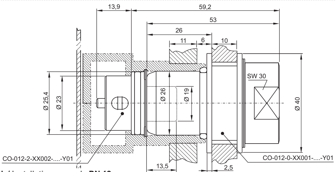
Einbaubeispiel / Installation example DN 12
