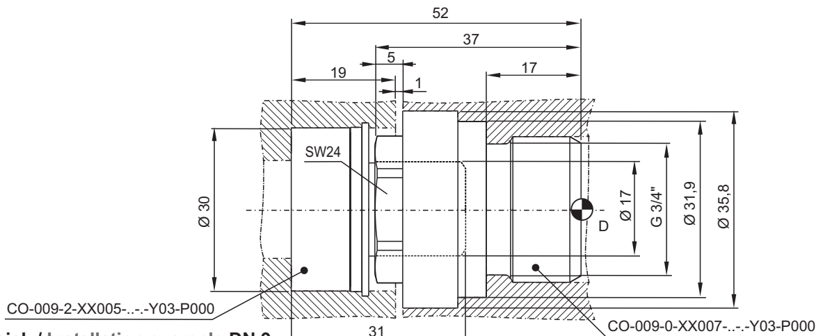
Einbaubeispiel / Installation example DN 9
