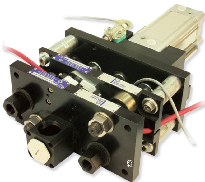
Sensor überwachte Multikupplung Sensor controlled multi coupling
