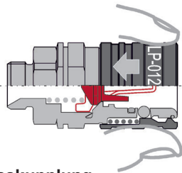
-0- Verschlusskupplung = Kupplung mit Ventil
