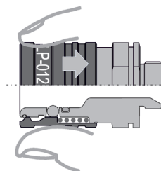
-4- Durchgangskupplung = Kupplung ohne Ventil
