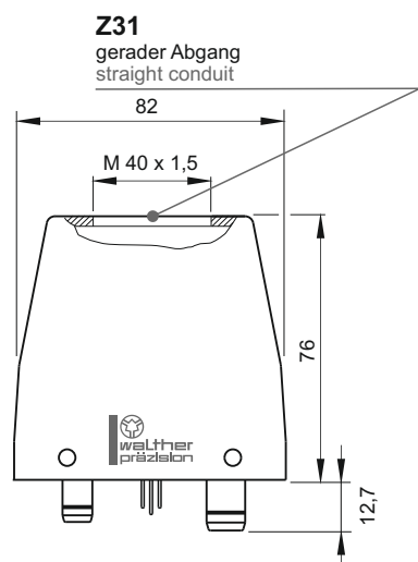
Loshälfte / free half 90410-1-...
